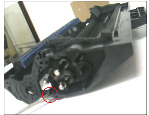
18. Para retirar la placa de soporte del rodillo primero destrabar el clip debajo del eje del rodillo de revelación.
