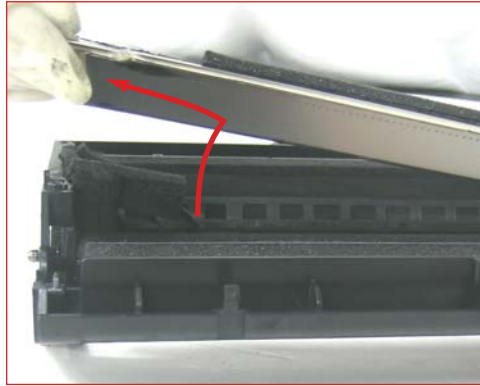
14. Levantar la cuchilla y deslizarla como se muestra:
