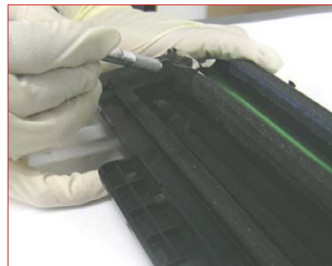
12. Seguir los pasos 12-14 y 22 si se reemplaza o se reinstala la cuchilla dosificadora. Estos pasos pueden omitirse si no se va a reemplazar la cuchilla dosificadora.
