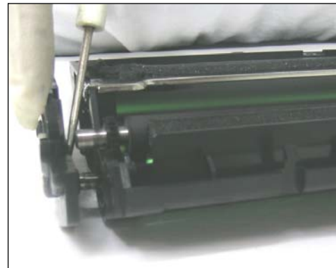
6. El lateral debe deslizarse suavemente. Si no, utilizar un pequeño desarmador plano para ayudar.
