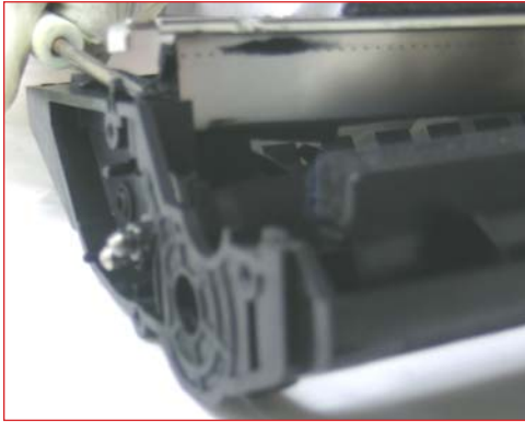
13. Una vez separado el sello se puede sacar la cuchilla dosificadora.
